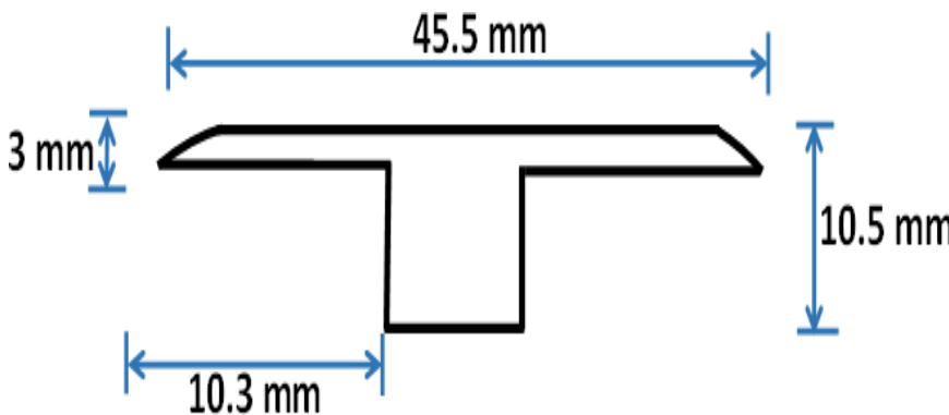
LAMINE MOULURE EN T (RECOUVREMENT)
