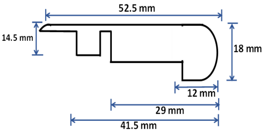
LAMINE NEZ DE MARCHE (RECOUVREMENT)
