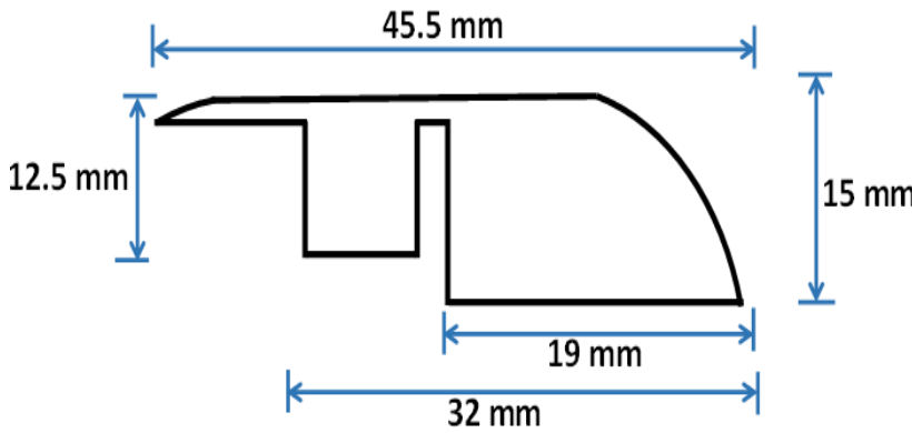
LAMINE RÉDUCTEUR (RECOUVREMENT)
