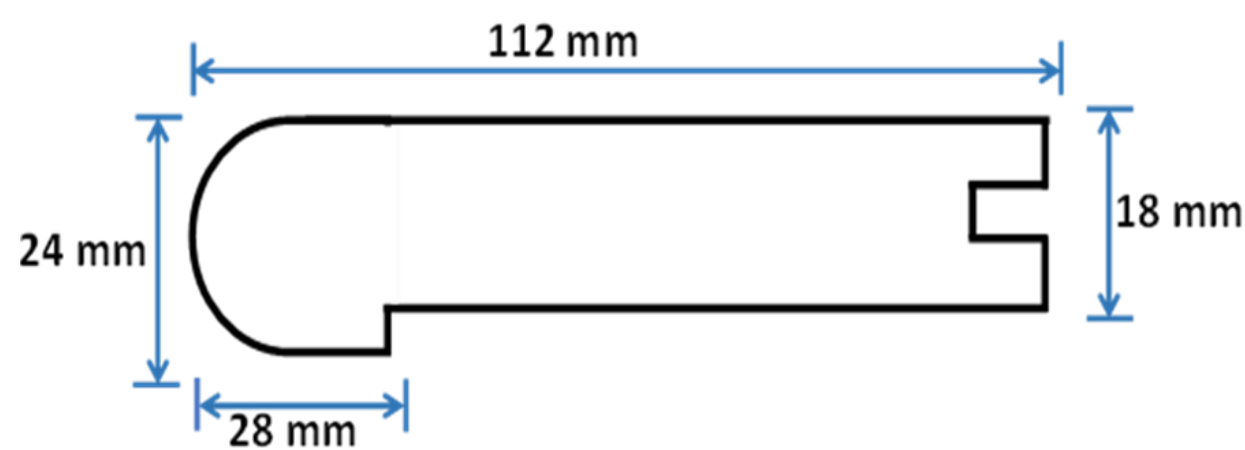
ENG HWD STAIRNOSE(FLUSH)
